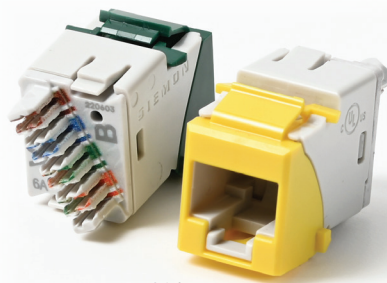
Keystone 插座
